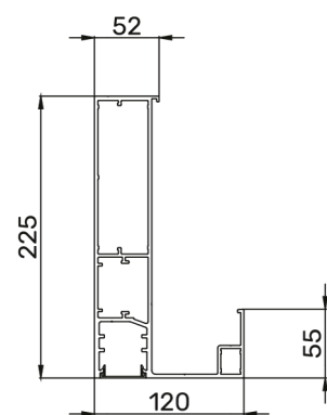
NOSNÍK
