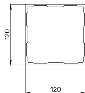
STĽP
